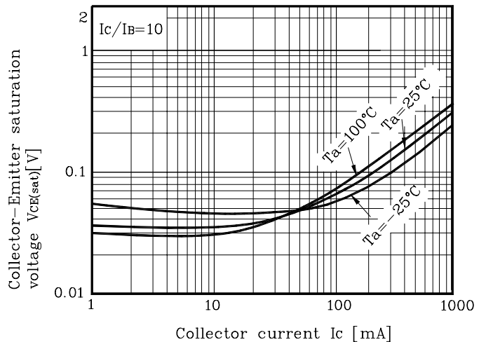
Fig. 4 V_{CE(sat)} - I_C
