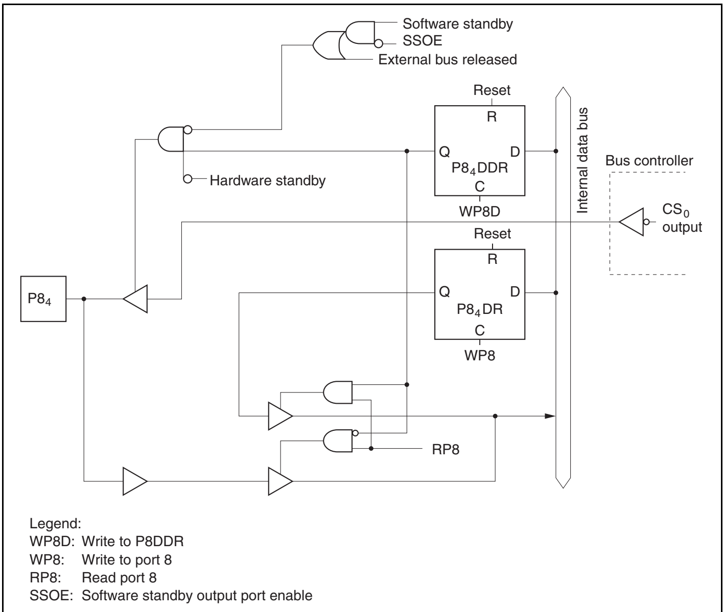
Figure C.4 (d) Port 8 Block Diagram (Pin P8 4 )
