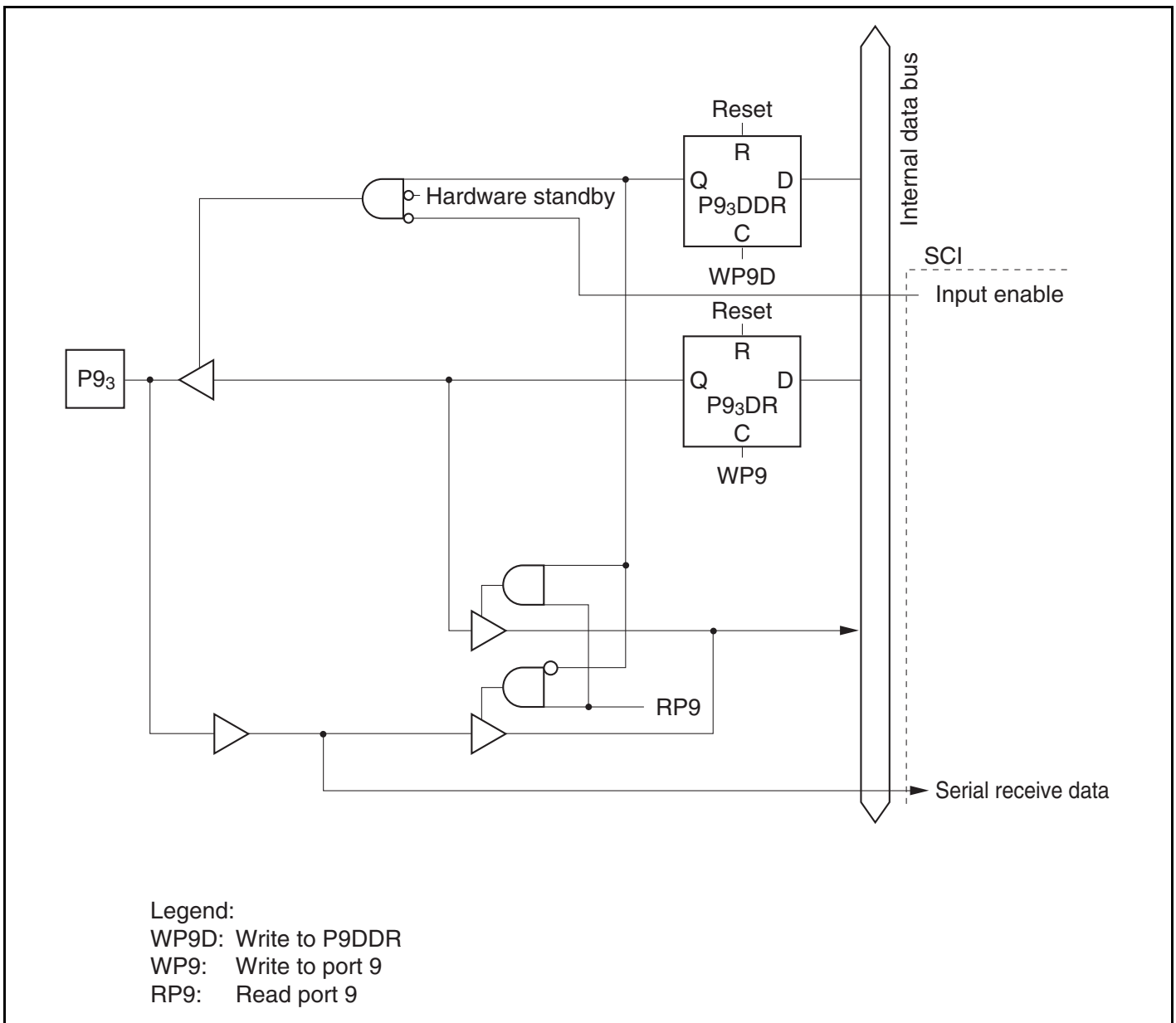
Figure C.5 (d) Port 9 Block Diagram (Pin P9 3 )
