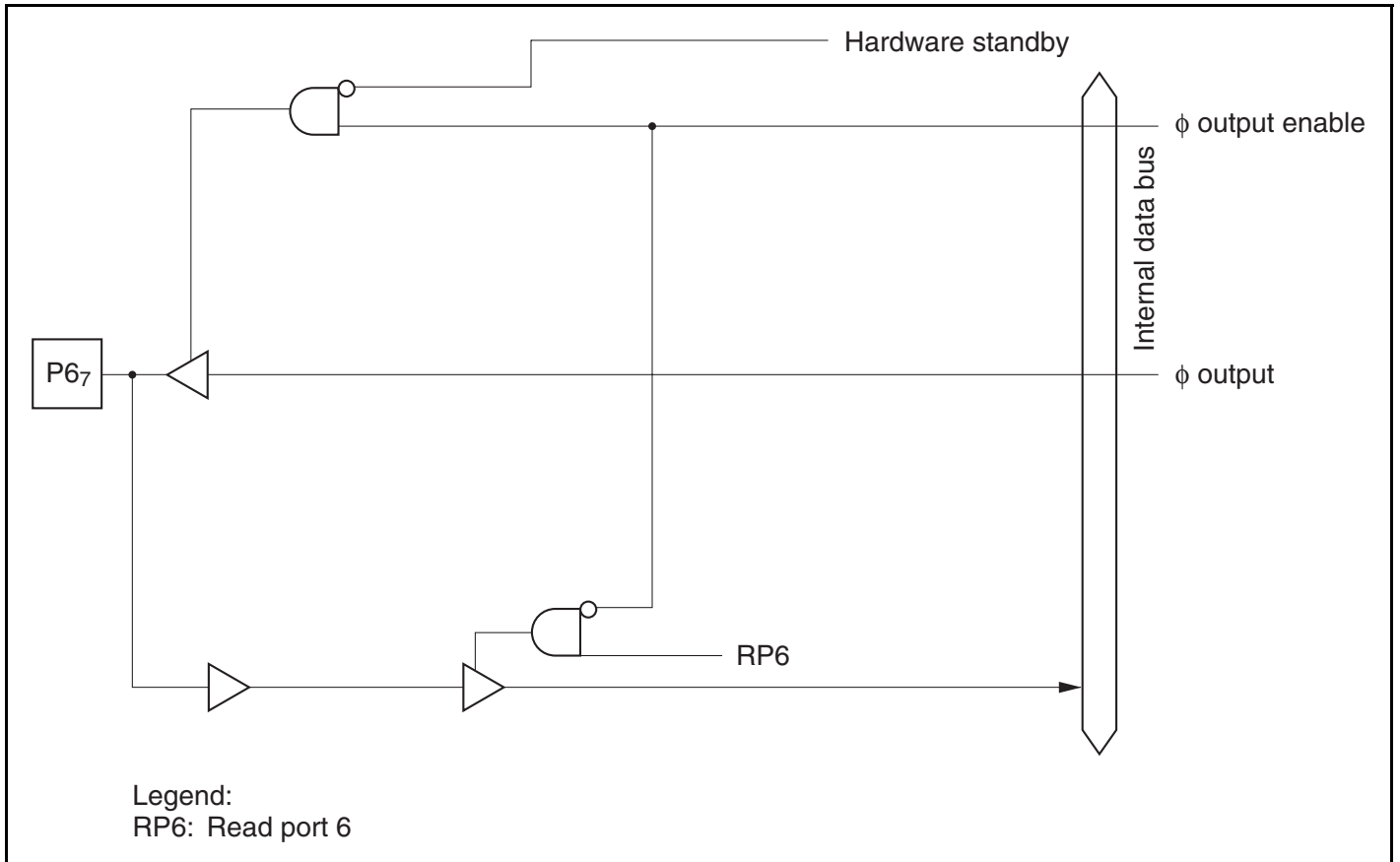
Figure C.2 (d) Port 6 Block Diagram (Pin P6 7 )
